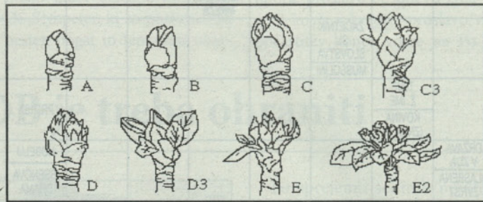
Slika 2: Skala razvojnih faz jablan po Fleckingerju
