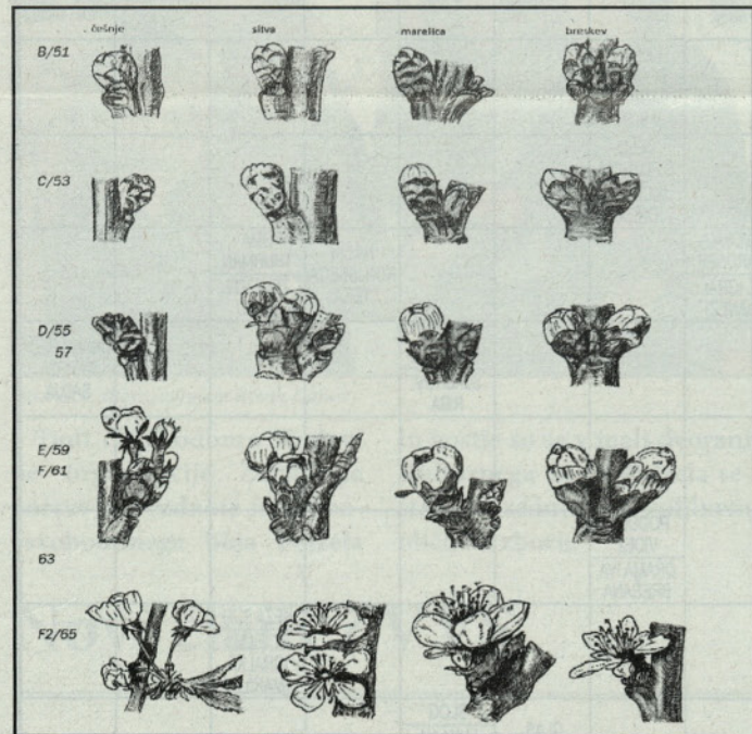
Slika 1: Skala razvojnih faz koščičarjev po Fleckingerju
