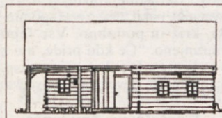
HIŠA V RISBI - Tehnični posnetek obstoječega stanja hiše (risal: P. Golob, Arhiv ZVNKD Novo mesto).
