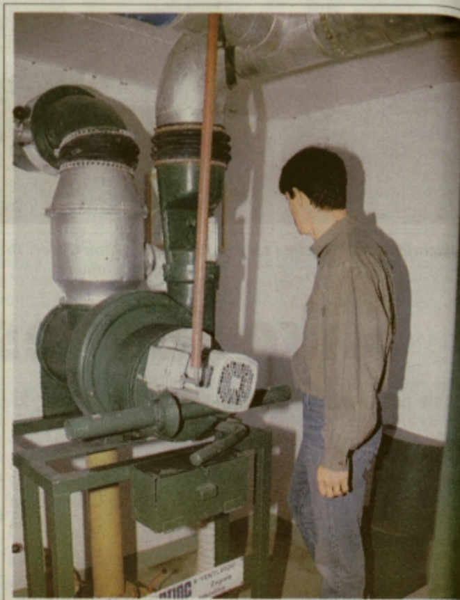
Vzdrževan prezračevalni sistem v enem od celjskih javnih zaklonišč, ki mu do popolnosti manjka le še filter za čiščenje zraka.
