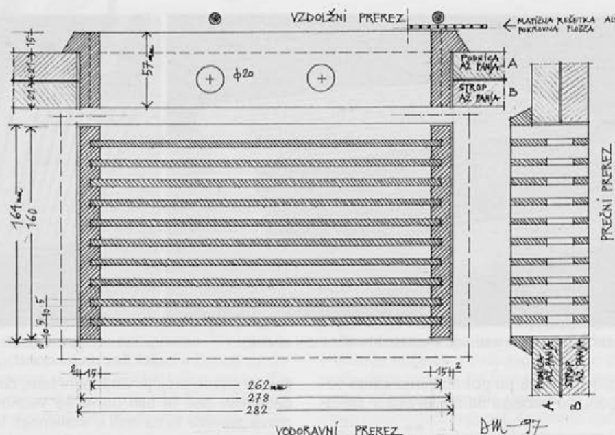
Lesen lamelni distančni vložek: načrt za izdelavo. Za navpično povezavo (združitev) AŽ panjev. Vložek vstavimo v izrezano odprtino (veho) na dnu in stropu panjev v skladanici. Avtor: dipl. inž. arh. Marjan Debelak.
