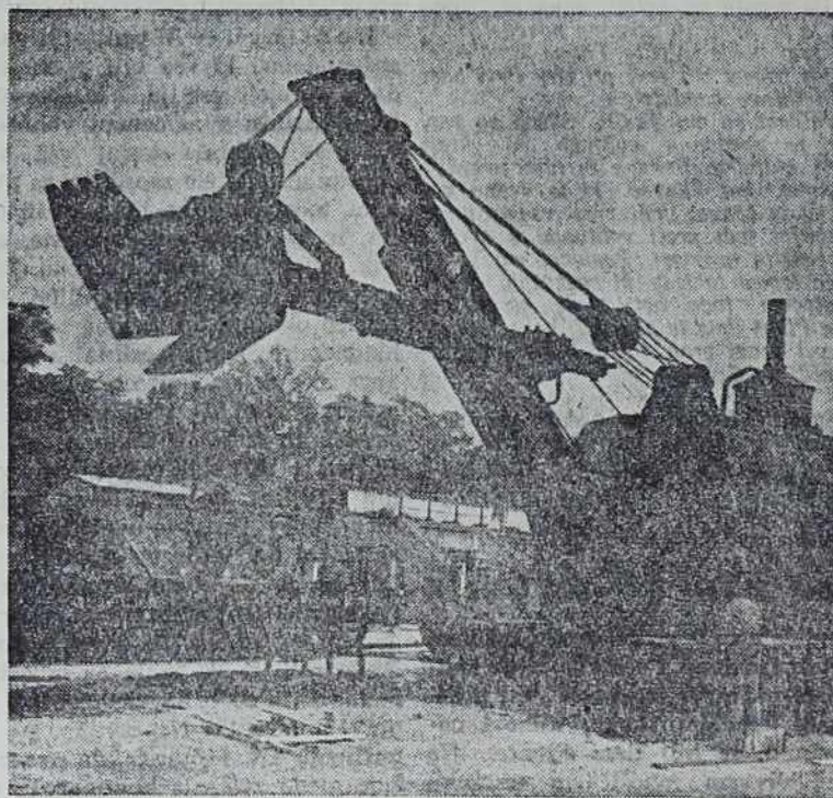
Veliki parni bager — ponos delovnega kolektiva tovarne »Djuro Djakovič«. Ta bager v 20 minutah izkoplje in naloži 1 vagon premoga. Uporablja se tudi za gradbena dela. Z njim ravna le dva človeka
