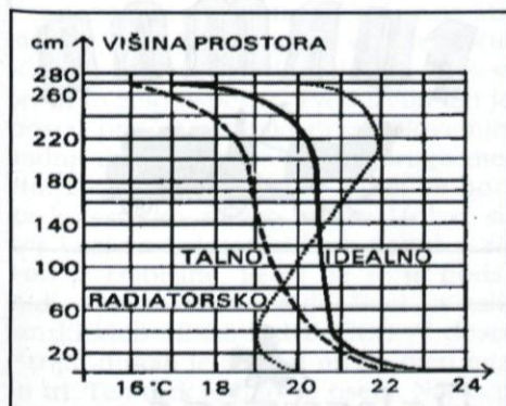
Sl. 1 Temperaturni vertikalni profil v prostoru pri različnih ogrevanjih
