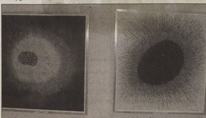
Veberičevi sliko Otrok vesolja in Oko vesolja.
