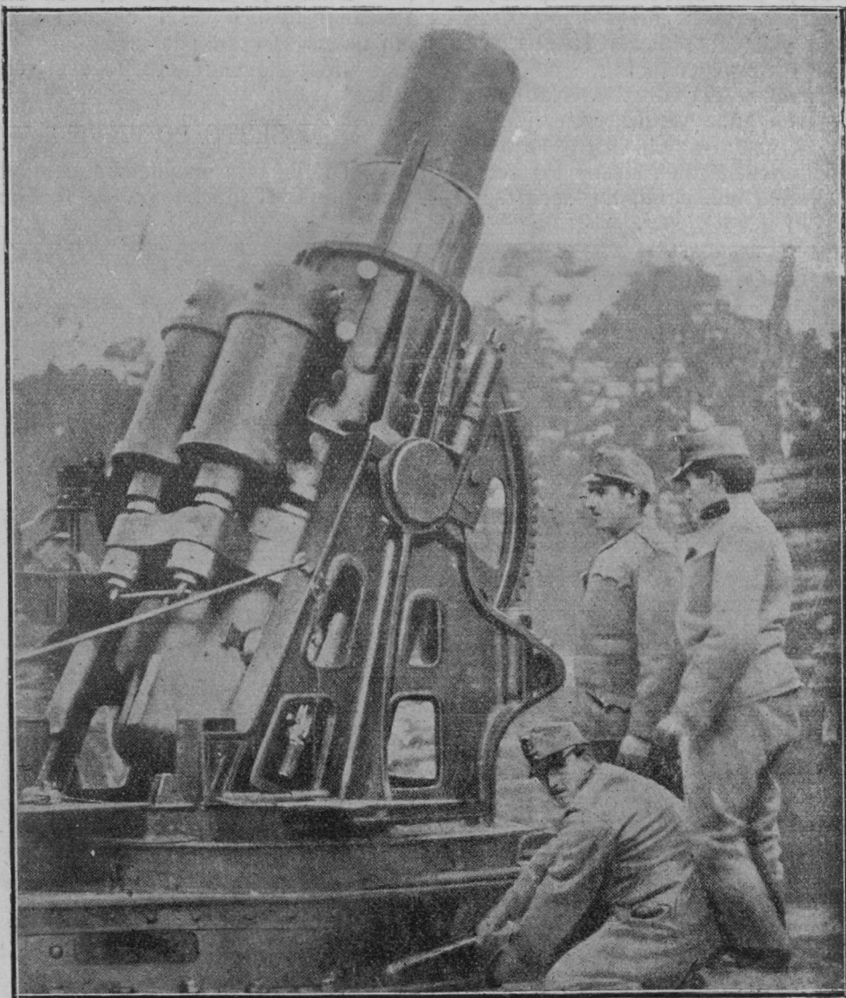
Možnar kalibra 30,5 cm, pripravljen za strel.
