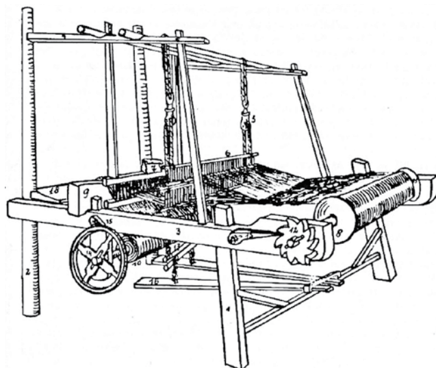
Sl. 43. Škatnikove statve, Gornji grad št. 119 (shema,ična risba). Legenda: 1 koza, 2 navpična stebrašča, 3 ojnica, 4 ostrešje, 5 knobe, 6 grebeni, 7 žlage, 8 prvi pom s šajbama, 9 zadnji pom, 10 spodnji pom, 11 šajba, 12 oven, 13 rigl, 14 kolo za šponanje, 15 rigl na kolesu za šponanje, 16 podnožjak ali nogavnica, 17 vage, 18 klop.
