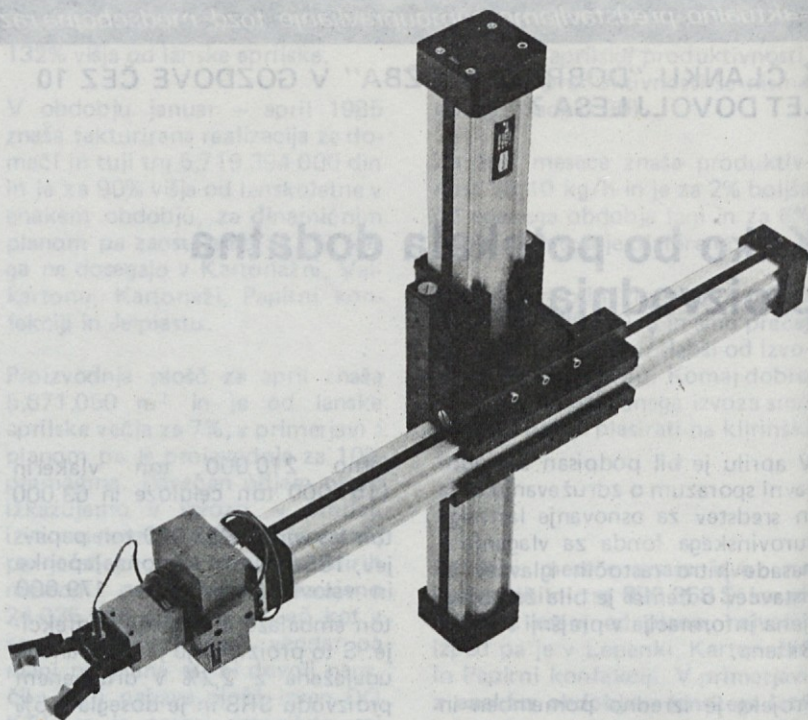
Primer enostavnega robota sestavljenega iz dveh pnevmatskih cilindrov brez batnice in rotirajoče prijemne glave
