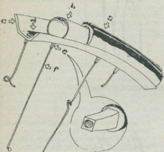
Slika 1. Prerez zračnice
