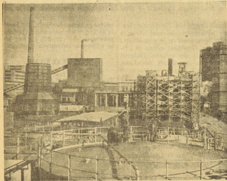
Koksarna v Lukavcu je poslala železarnam prvo pošiljko domačega koka
