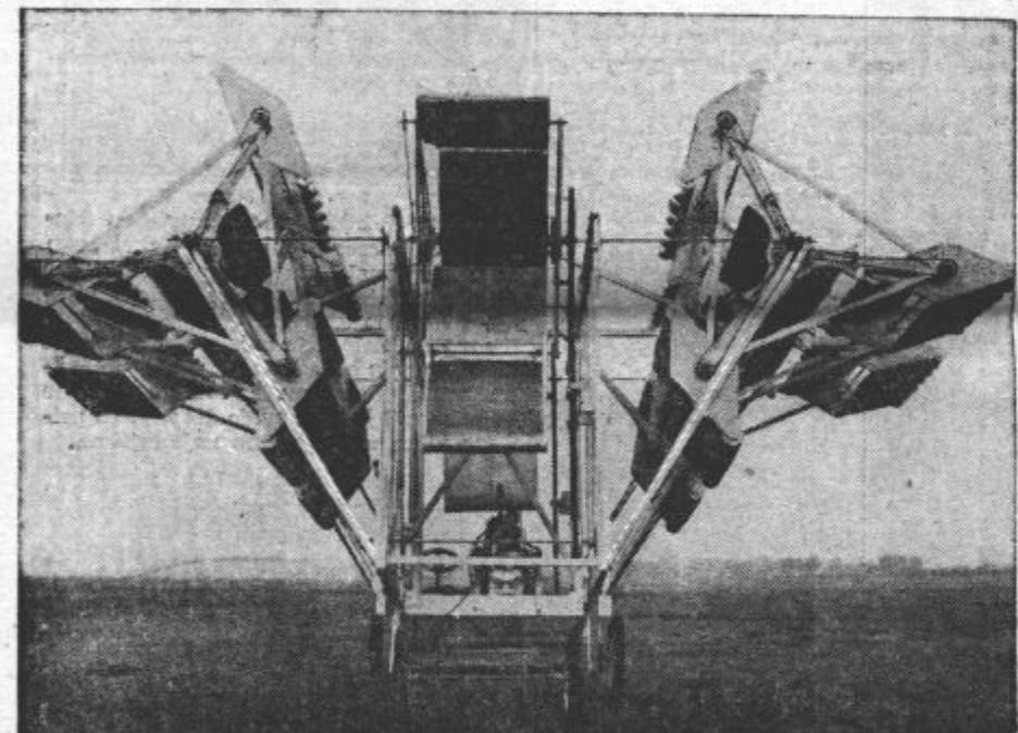
LETALO BODOCNOSTI. Pri New Yorku delajo poskuse z novo letalsko pripravo. Izumitelja sta zgradila nov tip letala, ki se dvigne v zrak navpično z zemlje in vsak čas lahko obstane v zraku na mestu. Naprava meri 6 m v višino in 8 m v širino
