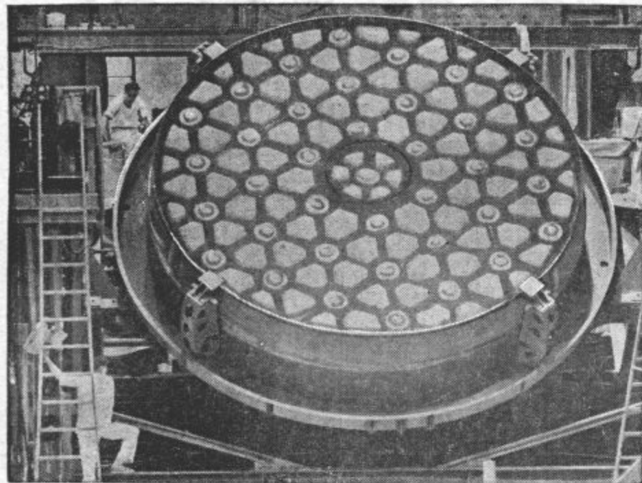
NAJVEČJI DALJNOGLED NA SVETU. Slika nam kaže ogromno zrcalo s premerom 6 m, ki ga sedaj montirajo v novi daljnogled v opazovalnici na Mountu Palomarju v Kaliforniji
