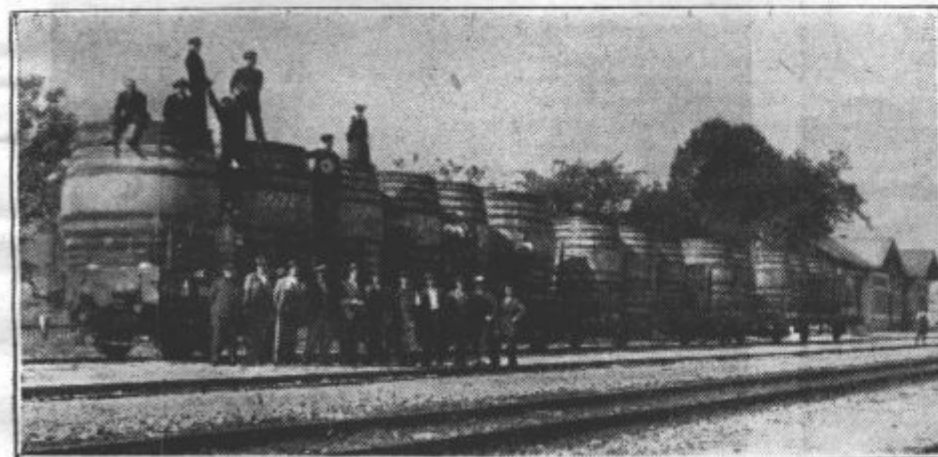
SODI IZ TACNA POD SMARNO GORO. Sodarška zadruga v Tacnu je izgotovila v zadnjem času že preko 60 sodov-velikanov za vsebino 1200 hl, in sicer za razne vinarske zadruga. Ta zadruga je prva v državi, ki izdeluje tako velike sode. Sodi so ovalni in okrogli. Gornja slika kaže sode, naložene na železniških vozovih na postaji v št. Vidu-Višmarjah. Spredaj stoje sodarski mojstri z načelnikom Ivanom Medvedom in svojimi pomočniki. — Sodi so zares strokovnjaško in odlično izdelani, da jih je ljudstvo kar občudovalo, ko so jih vozili na postajo. Sodi omenjene zadruga so bili tudi razstavljeni na državni obrtni razstavi ter so bili prodani vinarski zadrugi Bečevo-Niš. Tako je dobila sodarska zadruga v Tacnu popolno priznanje za odlično delo, kakršnega ne zmore kmalu kako drugo sodarsko podjetje izven Slovenije
