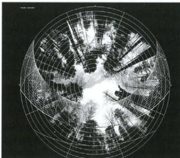
Primer posnetka z vrisanimi preslikavami poti sončevega sevanja (Čater, 2004)
