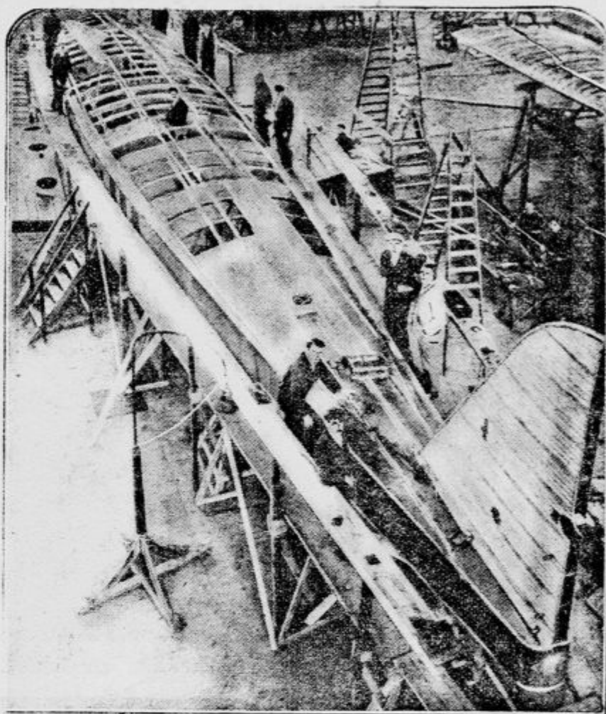
Trup hidroplana-velikana »Superwal«
