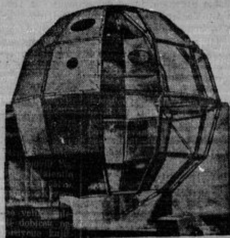
Polet v stratosfere nameravata podvzeti dva mlada avstrijska inženjerja Teodor Zichy in Braun. Slika predstavlja gondolo, ki ima obliko krogle in je sestavljena iz duraluminija.
