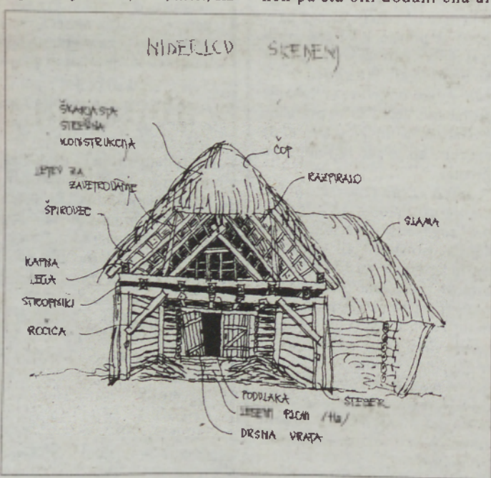
Niderlov skednji (avtorica risb Simona Kosi - Križnar, dipl. inž.)
