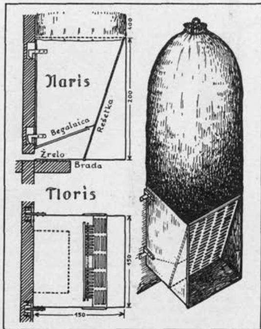
Freudensteinovo avtomatično prestrezalo za roje.
