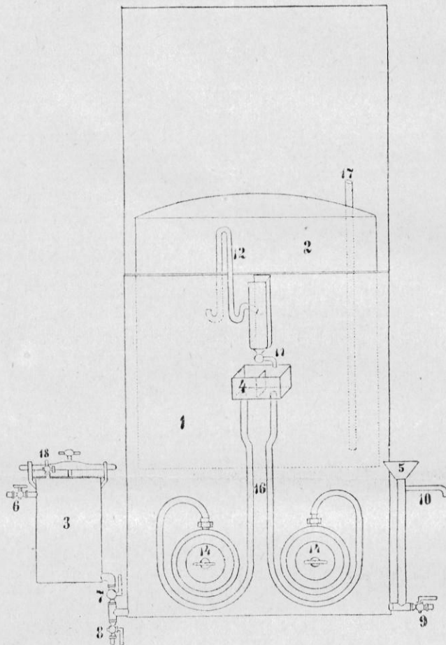
Pod. 12. Priprava za pridobivanje acetilena iz karbida.
