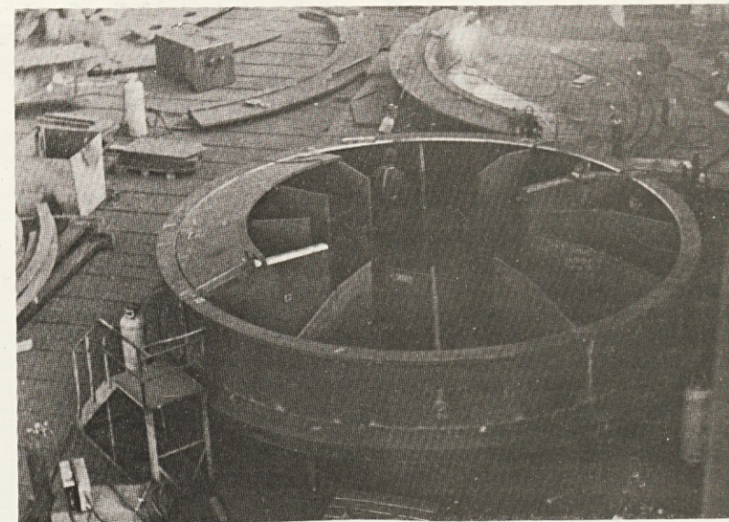
Sestavljamo prvega od šestih turbinskih pokrovov za HE HADITHA. Zvarjenec je iz dveh delov in je težak 90.787 kg. Na njem lahko varimo samo ročno elektroobložno, ker zaradi velike teže ne moremo uporabiti pozicionerja.
