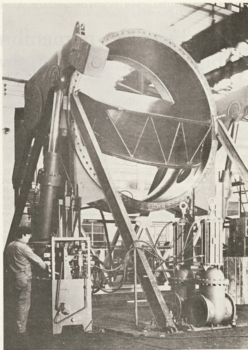
Vodostansko loputo (premer 4100 mm) za RHE Obrovac smo v celoti izdelali in jo tudi funkcijsko preizkusili v naši delovni organizaciji. Na fotografiji je vodostanska loputa med funkcijskim preizkusom.
