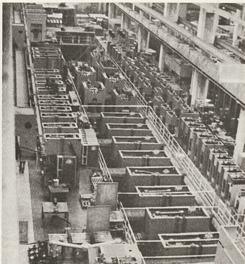
Montaža hidravličnih vlečnih strojev HVO-2-250 za SZ. Čas izdelave od lansiranja 11 mesecev, obdelava in montaža 3 mesece. (Foto: Silvo Belcijan).
