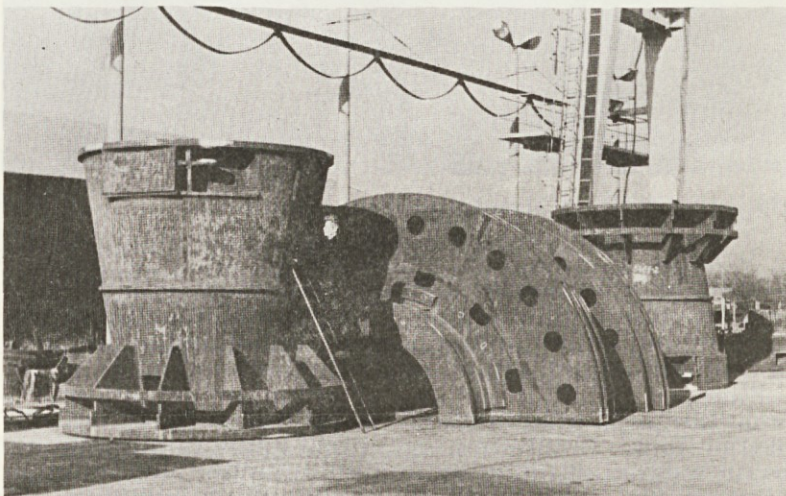
Zvarjenci za HE MAVČIČE na skladišču zvarjencev, kjer čakajo na nadaljnje operacije.
