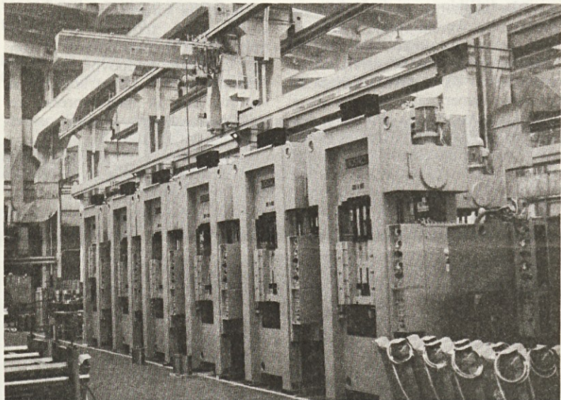
Hidravlični vlečni stroji HVO-2-100 za SZ. Čas izdelave od lansiranja 12 mesecev ali 3 mesece od obdelave in montaže. (Foto: Jolanda Jereb).
