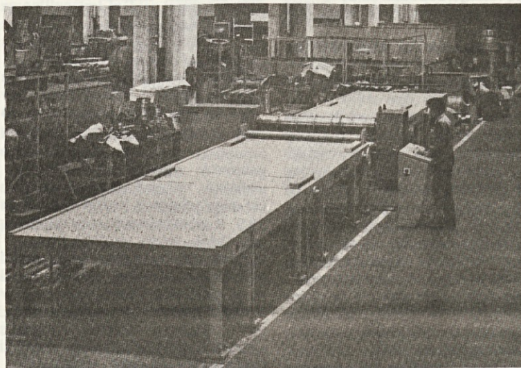
Pogled na montažo linije MPRT-1600/6 za Vozila Gorica. (Foto: Jolanda Jereb).
