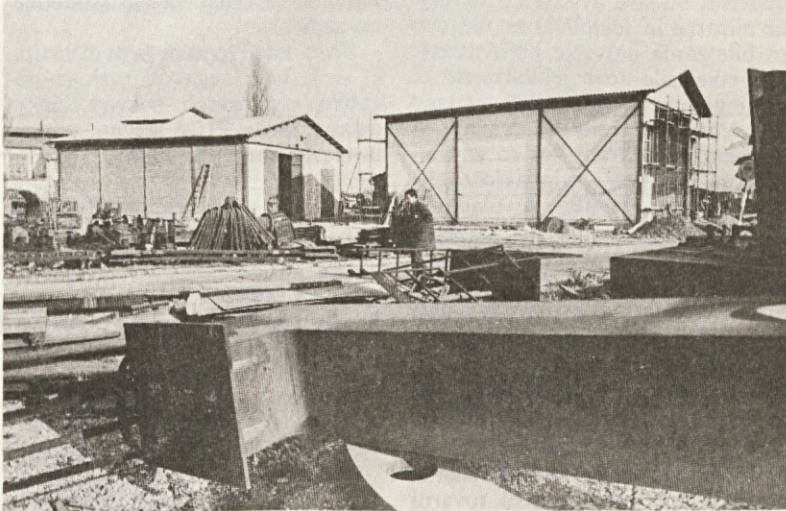
Rekonstrukcija peskarne in barvarne. TOZD PZO je sodeloval s ključavničarskimi deli pri postavitvi konstrukcije za barvarno in obnovitvi konstrukcije peskarne. V rekonstruirani peskarni bomo peskali samo z jeklenim zdrobom, kar je potrebno zaradi boljše površinske zaščite zvarjencev.
