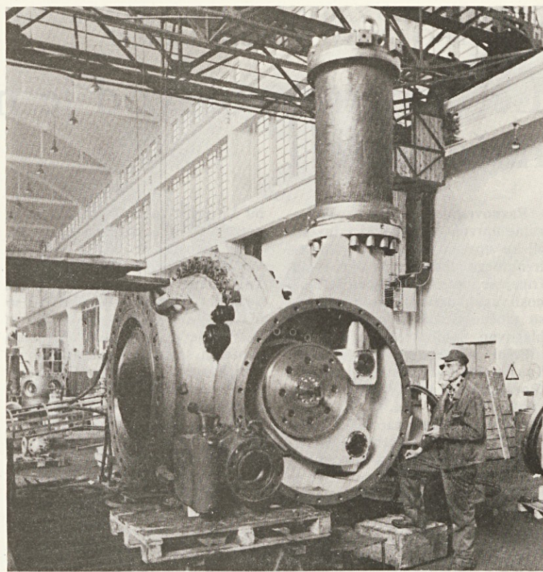
Kroglasti zasun za hišno turbino HE Peručica, je bil eden prvih, ki smo jih pred 28 leti izdelali v Litostroju. Ima premer odprtine 200 mm in je težak približno 100 kg. Pred kratkim je bil pri nas v generalnem remontu. Na fotografiji ga lahko primerjamo s 76-tonskim kroglastim zasunom za RHE Obrovac. (Foto: T. Š.)
