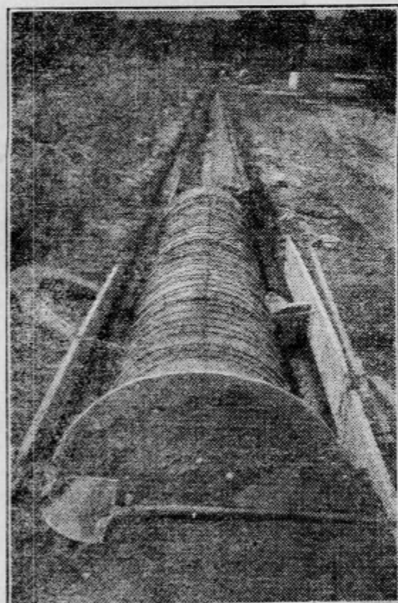
Betoniranje velikega kanala
