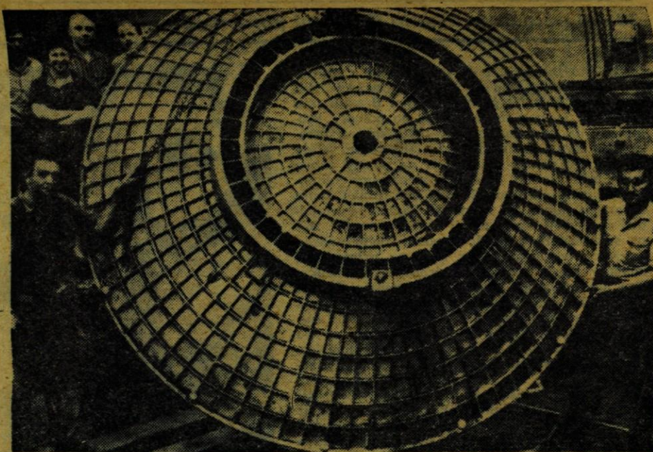
V Franciji v bližini mesta Menton so zgradili aluminijasti reflektor, ki bo zbiral podatke iz umetnih satelitov v vesolju. Reflektor tehta več kot eno tona.
