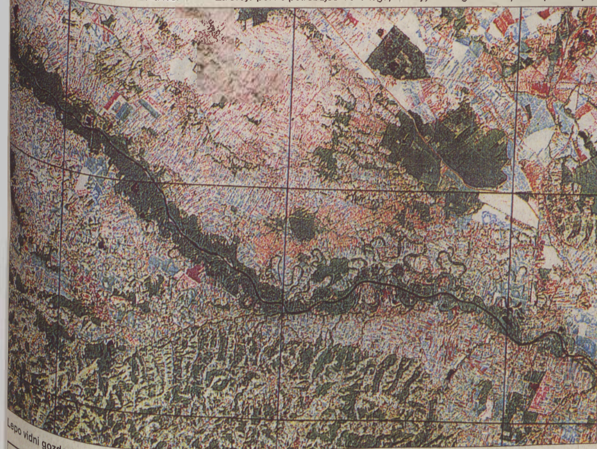
Lepo vidni gozdovi v nižinskem delu Prekmurja in obmurskem pasu - satelitski posnetek
