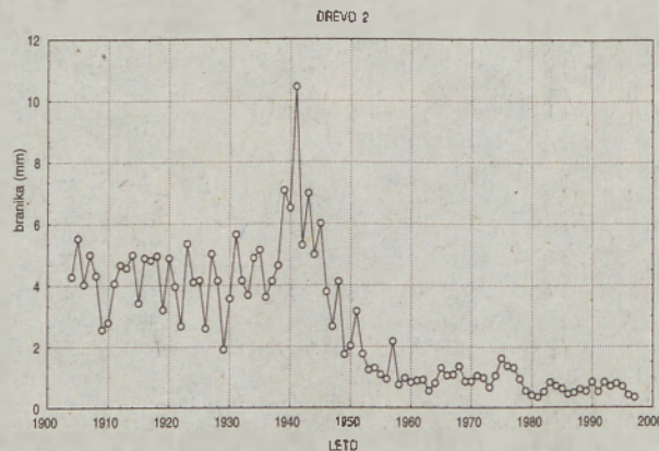
Graf št. 1: Padec debelinskega prirastka po prvih melioracijah reke Ščavnice leta 1956
