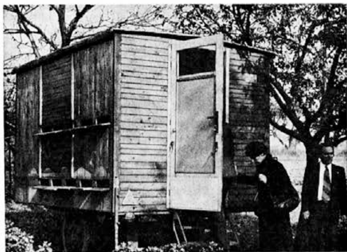
Enoosna traktorska prikolica za 20 panjev. Foto: avtor
