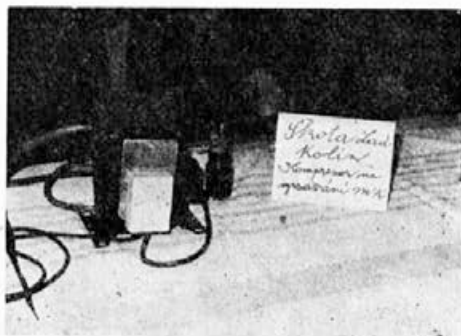
Kompresor hladilnika uporabljen kot sesalnik za matični mleček. Foto: avtor
