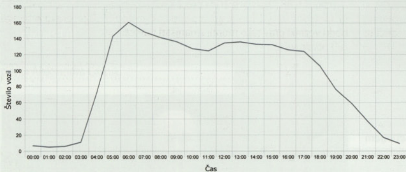
Graf 3: Gostota prometa glede na čas dneva.
