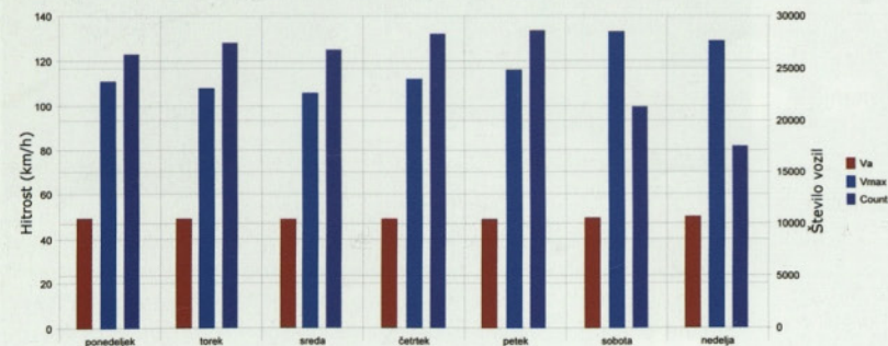
Graf 4: Statistični podatki glede na dan v tednu.
