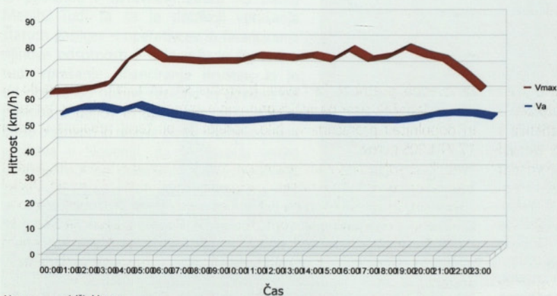
Graf 1: Hitrosti glede na čas dneva.
