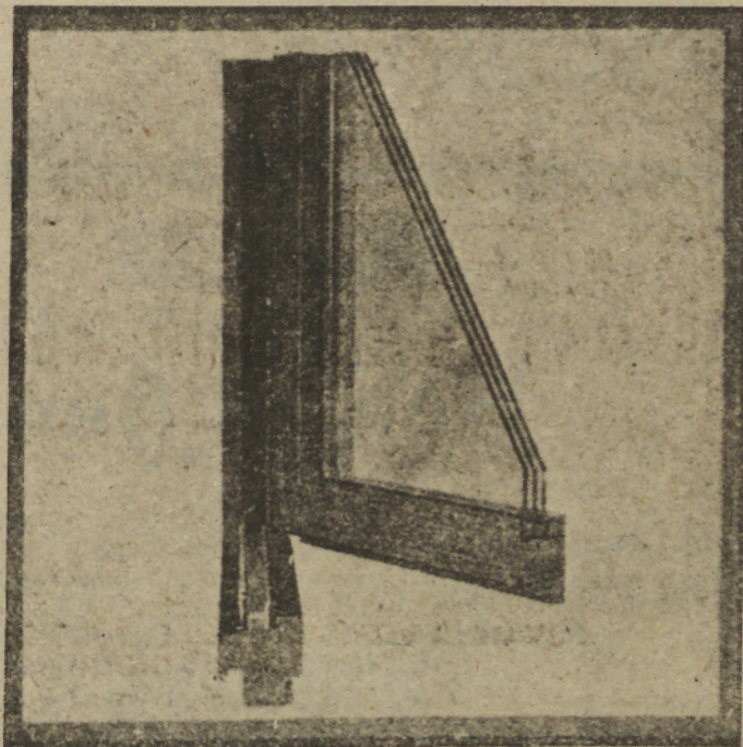
OKNO IZOPLUS ZASTEKLENO S TRISLOJNIM IZO STEKLOM — PREREZ
