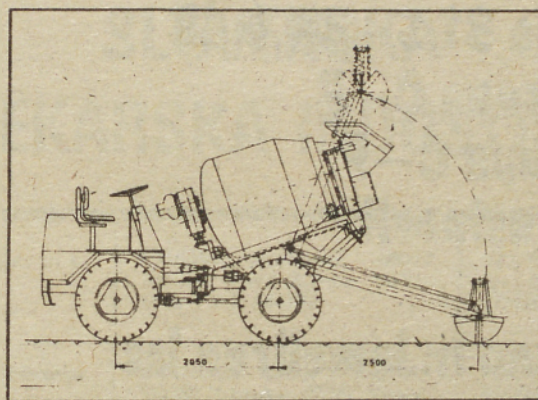
MOBILNI MEŠALEC BETONA MM 1000 , ki lahko vozi po najtežjem terenu.
