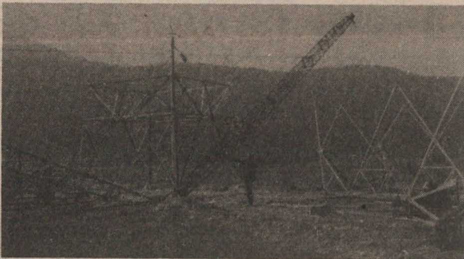
Sestavljanje jeklene konstrukcije na stebri 50 pri Strahomerju
