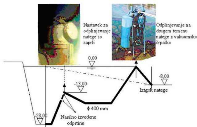
Slika 4 • Shema zahodnega kraka natege z mesti nasilno izvedene odprtine, s katerimi so natege onespobili ((Rismal, 1999), (Rismal, 2004), (Rismal, 2011)).
