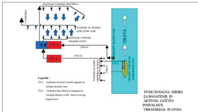
Slika 31 • Koncept povečanja črpalnišča na Vrbanškem platuju z obrežnim filtratom Mariborskega otoka in levega brega Drave na 700 l/s (Rimal, 2015).
