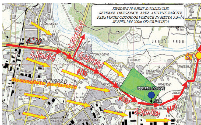
Slika 32 • Z dragim, 5 km dolgim cevovodom Ø180 iz duktilne litine za 5,3 m³/s padavinskega odтока iz celotne obvoznice mimo vodarne ljubljanskega vodovoda v Hrastju, 200 od vodarne, je varnost črpane podtalnice dodatno ogrožena (Rimal, 1999).
