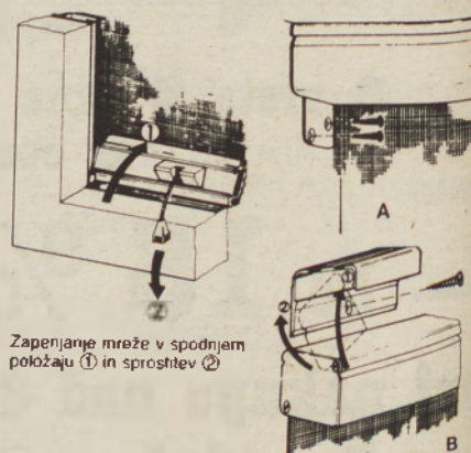
Prikaz bočne pritrditve KOMARNIKA P in zaskočna pritrditev KOMARNIKA R
