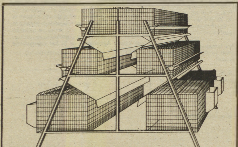
Trietažna baterija s Hobby. Namenjena je ljubiteljem in rejcem. Spodnja etaža je za samice, srednja za odstavljenke, zgornja pa za pitance. Delo in čiščenje je enostavno, baterija pa omogoča tudi dober pregled nad živalmi. Baterija je kot enostranska (dve samici s pomladkom) ali dvostranska (štiri samice s pomladkom). Dimenzije: 194 (97) x 85 x v. 170 cm.
