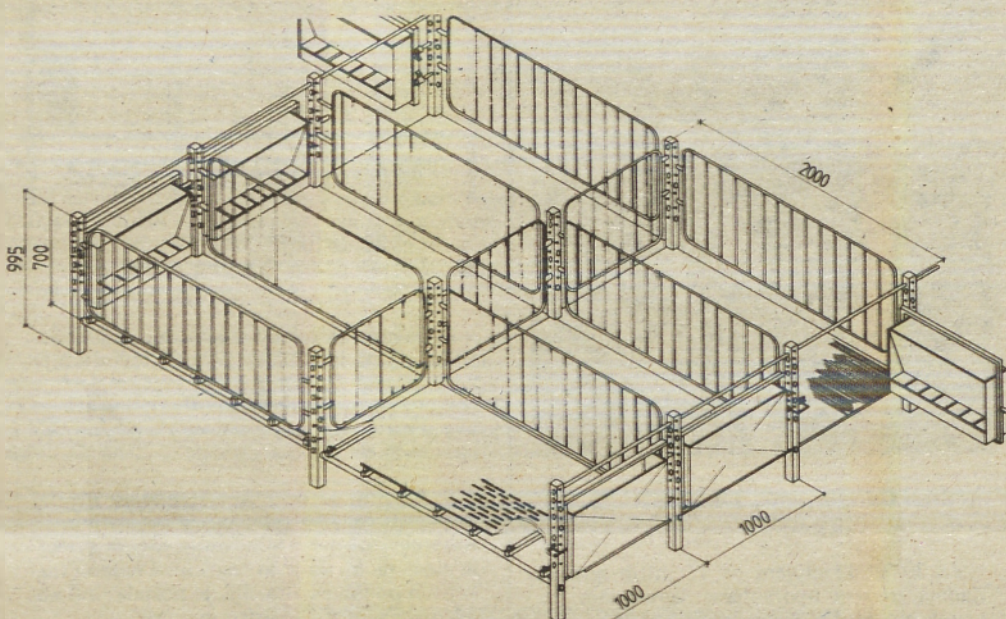
Boks za pujske (do 25 kg). Dimenzija: 2000 x 1000 x 995 mm, sestavni deli: nosilni montažni stebri, tla KOTERM, plastika ali perforirana Al-pločevina, bočne rešetkaste stranice, vrata z vgrajenim hranilnim prostorom, avtomatski napajalnik.
