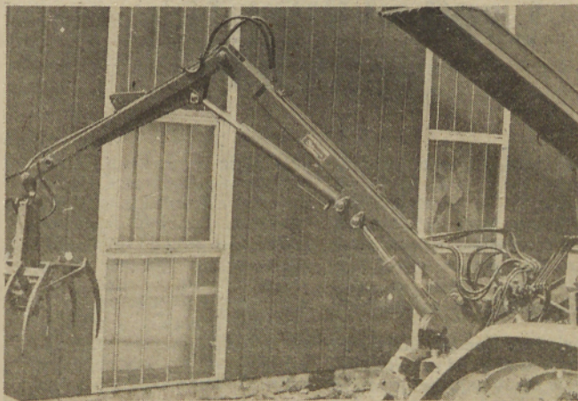
Nakladalec gnoj, izdelek soboškega Agroservis
