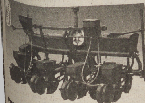
Pnevmatska sejalnica za koruzo.
