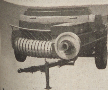
Pobiralna stiskalnica za seno in slamo.
