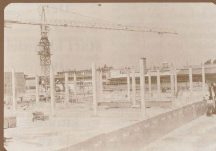
Postavljanje nosilnih stebrov na pilote
