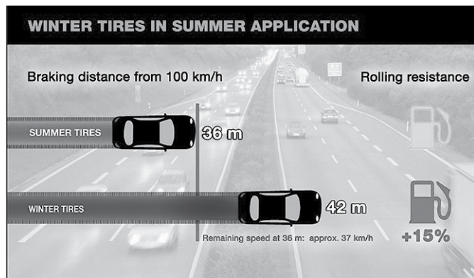
Prikaz razlike v delovanju zimskih in letnih pnevmatik na razgretem asfaltu
