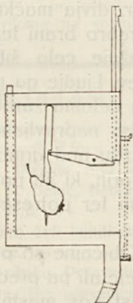
Slika C. Podolžni prerezní prikaz nastavljene skrinjice, ki učinkuje na pritisk.
