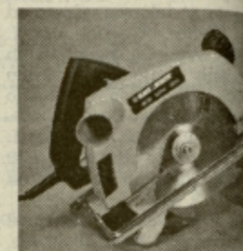
krožna žaga, BLACK&DECKER, BD 50, 1020 W, globina do 62 mm, premer 184 mm
