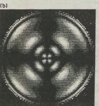
(a) kaže intenzitete za kroglo s polmerom R = 3,5 \mu\text{m} , (b) pa intenzitete za kroglo s polmerom R = 6,5 \mu\text{m} . Skupni podatki so: \lambda = 500 \text{ nm} , n_1 = 1,7 in n_2 = 1,5 .
