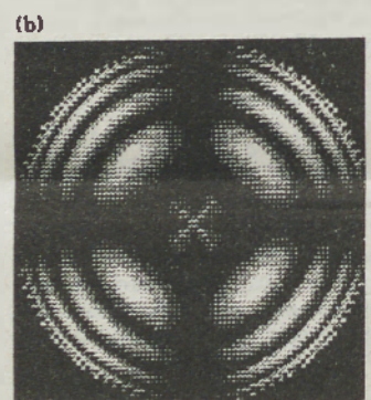
(a) kaže intenzitete za kroglo s polmerom R = 3,5 \mu\text{m} , (b) pa intenzitete za kroglo s polmerom R = 6,5 \mu\text{m} . Skupni podatki so: \lambda = 500 \text{ nm} , n_1 = 1,5 in n_2 = 1,7 . Svetloba se razširja v smeri osi z
