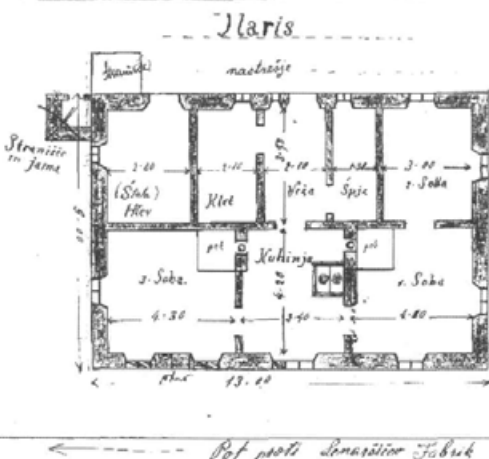
135. Orientacija Kodermanove hiše že sledi intimnejšemu načinu bivanja; v hišo se vstopa skozi vežo na dvoriščni strani in naprej v kuhinjo. Glavni prehod še vedno vodi preko cele širine hiše, ob strani so sobe, shrambe, klet, cestnega vhoda pa več ni. V vogalnem delu je hlev, ob njem zunanji straniščni prostor. Risal: Tesar Janez Lenarčič, Blatna Brezovica, 1931. Vir: ZALj, t.e. 4, a.e. 481.
