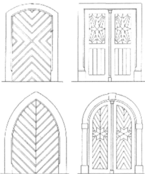
269. Primeri različno opaženih vratnih kril, kakor so sestavljali vratnice zlasti pred 19. stoletjem. Risal: F. Dobnik po Sičevi in Karlovškovi zbirki. Vir: Karlovšek 1939: str. 100, sl. 49.
