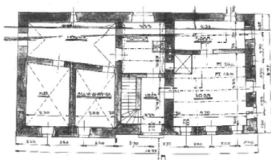
127. "Tlocrt" Hladnikove hiše, Verd 20. Zidovi, ki niso postavljeni pravokotno, nakazujejo verjeten razvoj stavbe - združevanje posameznih, prvotno manjših enot (stanovanjskega in gospodarsko shrambnega dela). Vhod v hišo je en sam - z dvoriščne strani. Risal: Ivan Petkovšek, Vrhnika, leto 1919. (Risba je poškodovana). Vir: ZALJ, t.e. 13, a.e. 1473.
