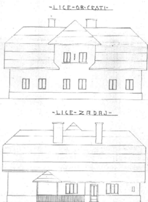
215. "Načrt za predelavo stanovanjske hiše" Franca Furlana. Risal: Alojz Jurjevčič, tesar, Vrhnika, 1941. Vir: ZALj, t.e. 2, a.e. 162.
