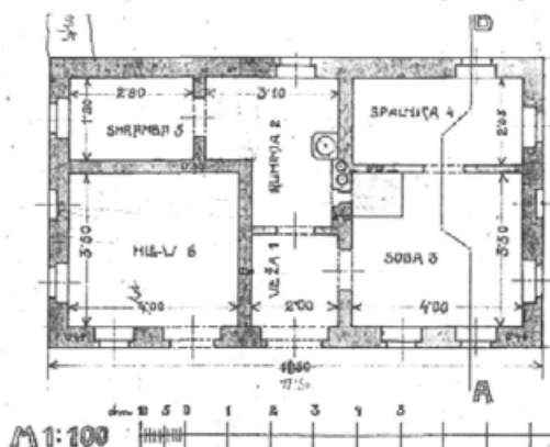
128. "Načrt pritlične hiše Gašperja Leskoveca v Vrdu." Skromnejši lastniki so prostor za kravico dobesedno vrnili v tloris doma. Tako je bilo prostora za vse dovolj, hiša pa je imela še vedno urejen vizez in enotno zasnovan tloris. Na mestu te hiše je danes tovarna LIKO. Risal: Zidarski pomočnik Fran Varšek, leta 1908. Vir: Lelik, t.e. 6. a.e. 655.
