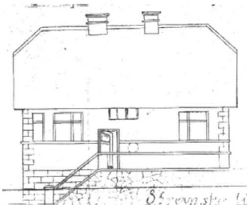
292. Na načrtu "za enodružinsko hišico g. A. Dobrovolca" leta 1932 je vrisano likovno pestro pročelje hiše; streha s čopi, mansardni balkon, šivani robovi in s fasadnim zidcem ločene etaže, rustikalno členjeno pritličje ... vhodna vrata, priprto narisana na stranski fasadi, pa so enokrilna. Risal: Zidarski mojster Gašper Petkovšek, Vrhnika. Vir: ZALj, t.e. 1, a.e. 114.
