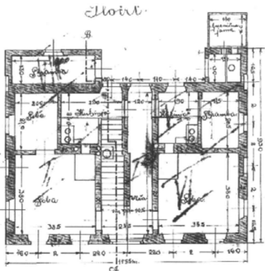
130. Hiša, ki jo je zgradil leta 1911 Janez Levč, ima od sprednjega obodnega do zadnjega dvorišnega vhoda speljan dolg hodnik. Kuhinji sta načrtovani dve, postavljeni ena nasproti druge, proti dvoriščni strani hiše. Hiša je do današnjega dne ostala skoraj nespremenjena in vzorno ohranjena. Risal: Ivan Petkovšek, 1911.
