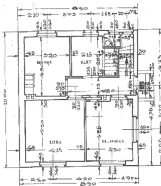
136. "Načrt enodružinske hiše za g. Janeza Japelc-a, čev. mojster Verd št. 9 na parc. št. 573." V stanovanjski hiši z mansardo je tudi čevljarška delavnica. Vhod v hišo je en sam – s stranskega dvorišča. Risal: Stavbno podjetje Stavbenik Furlan- Kunaver, Ljubljana, 1933. Vir: ZALj, t.e. 3, a.e. 307.
