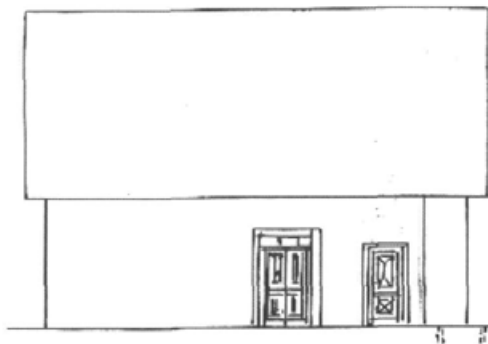
139. "Načrt enostanovanjske hišice za g. Marijo Pajsar, posestnico v Verdu." Vir: ZALJ, t.e. 8, a.e. 952.
