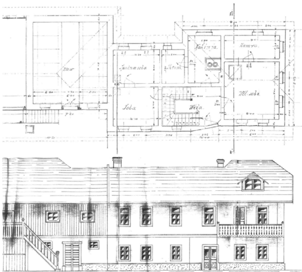
131. Načrt prezidave Mačkove hiše; tloris in pogled. Risal: Pernuš iz Kranja, 7. april 1922. Vir: Štefka Cunder
