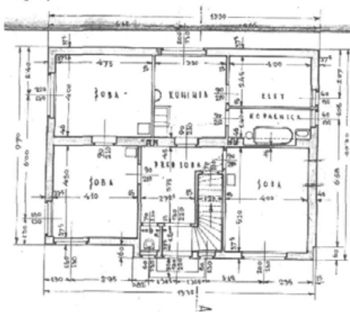
134. Rosenwirthova hiša je bila zgrajena leta 1932. Nove oblike hišne zunanosti v sebi še vedno skrivajo strukturo starejših stanovanjskih hiš, v katero se vključujejo tudi že načrtovani sanitarni prostori (stranišče, kopalnica). Hkrati pa stara prostorska zasnova ne sledi več novemu načinu bivanja, saj glavnega hišnega vhoda praktično ne uporabljajo in je težišče življenja na dvoriščni, zadnji strani hiše. Risal: Zidarski mojster Jakob Celarc, Vrhnika, 1931. Vir: ZALj, t.e.10, a.e.1102.
