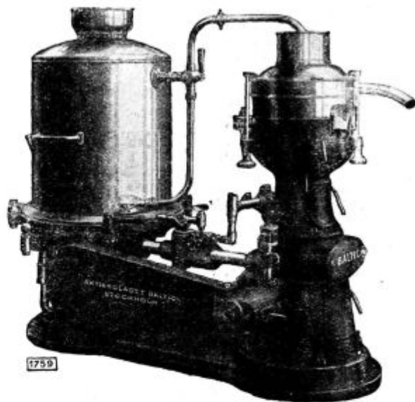
Pod. 34. Posnemalnik „Baltic“ na parno turbino z ogrevalnikom.
