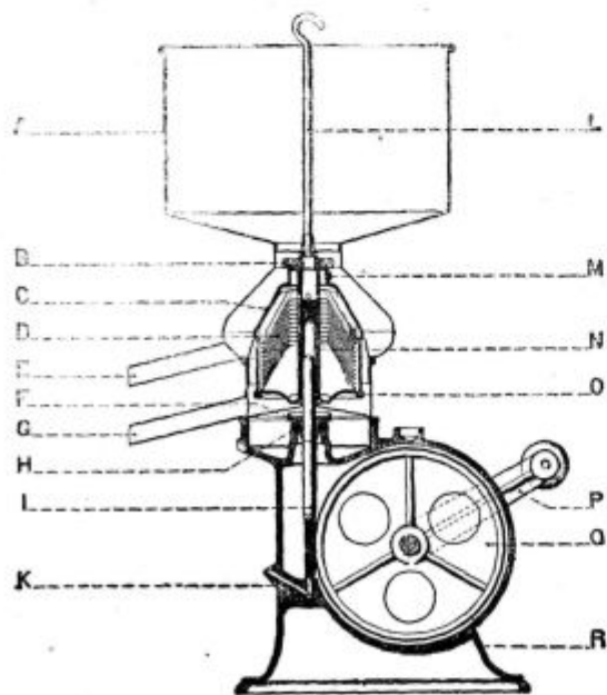
Pod. 33. Prerez posnemalnika „Baltic“.
