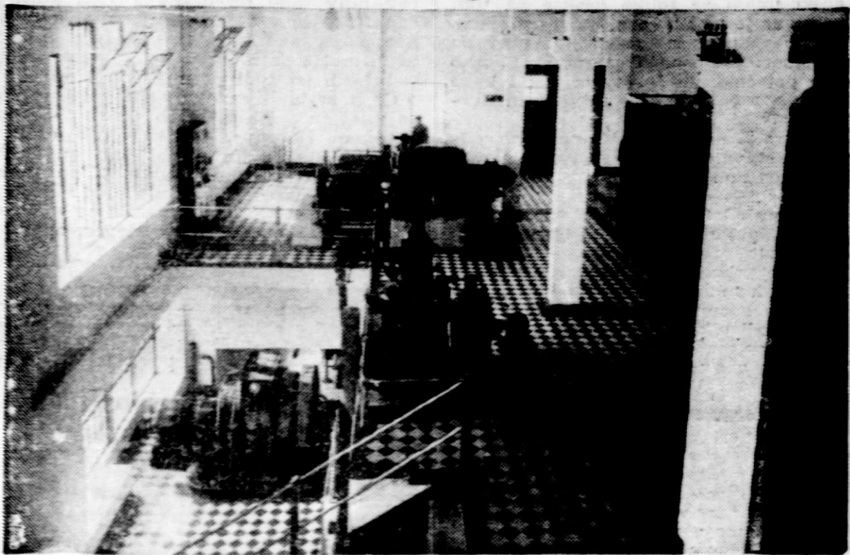
Največja domača zasebna elektrarna v dravski banovini. Oskrbuje pretežno industrijo in obrtništvo v Kranju, okolici in Medvodah. Sodeluje s Kranjskimi deželnimi elektrarnami in Elektrarno Škofja Loka d. d. v Škofji Loki.
