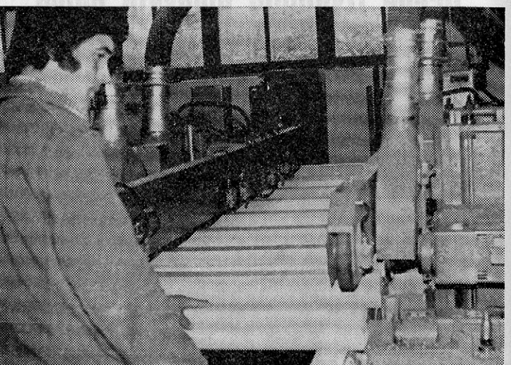
Obrezovalka v oddelku pohištva. Stroj ima na vsaki strani po sedem delovnih vreten. Upravljač stroja na njem lahko v enem postopku obžaga elemente na točno dolžino, nadalje zaokroži lamelo za pohištvo Dota, začepi prečko postelje in še vrsto drugih operacij
