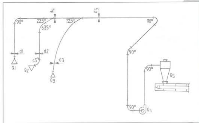
Slika 2: Shema odsesovalne naprave
