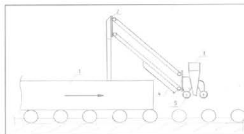
Slika 3: Skica sesalne šobe na konzoli
