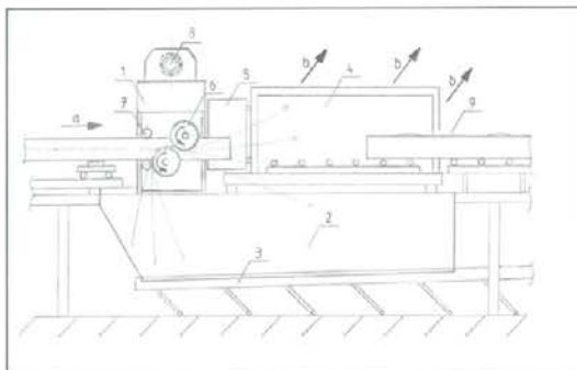
Slika 1: Notranji pogled na sklop žagalnega stroja
