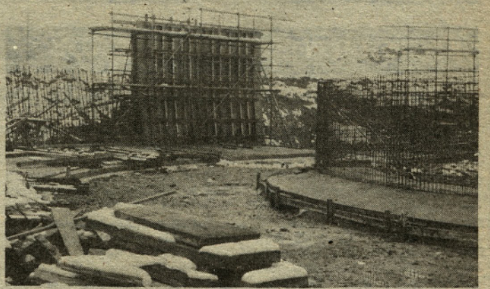
Prva faza osrednje čistilne naprave za odplake v Kasazah poteka skladno s terminskim planom. Izvajalca del Gradis in Nivo Celje zagotavlja, da bo čistilna naprava začela obratovati že jeseni. V teku je tudi izgradnja glavnega kanalizacijskega zbiralnika Kasaze-Žalec. Zavedajoč se, da je varstvo podtalnice in skrb za čisto okolje življenjskega pomena, zato tej dejavnosti namenimo tudi velik del sredstev.
