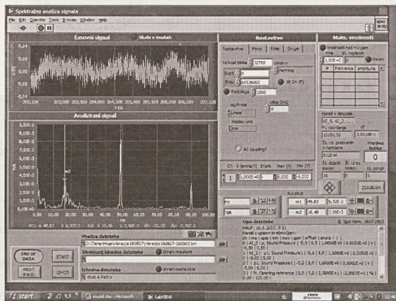
Meritev vibracij, ki jih povzroča nizkofrekvenčni hrup z izvorom v tovarni Lesonit. Meritev je bila opravljena 16.8.2007 ob 0321. Meritev kaže tri maksimume in sicer pri 16.5Hz, 49Hz in 90Hz.
