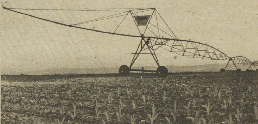
Sistem namakanja AGROPIVOT.
