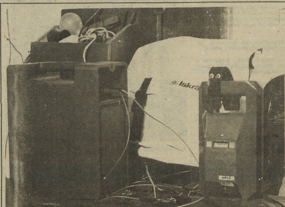
Priključitev električnega pastirja preko polnilnika baterij na omrežno napetost 220 V.
