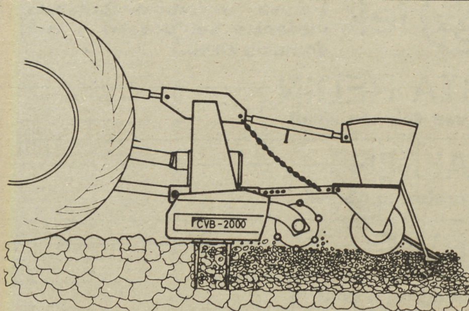
Kombinirana (sočasna) uporaba vrtavkaste brane CVB CIMOS s sejalcem.
