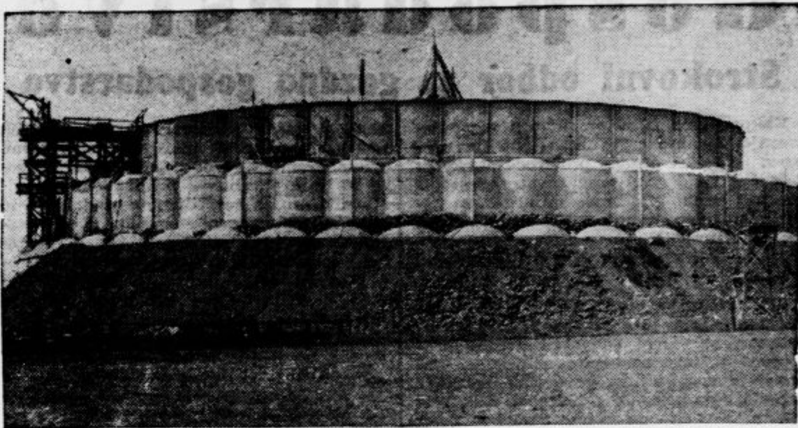
Ima mesto Nantes v Franciji. V njem je prostora za 40 tisoč kubičnih metrov voda. Rezervoar je zgrajen iz armiranega betona
