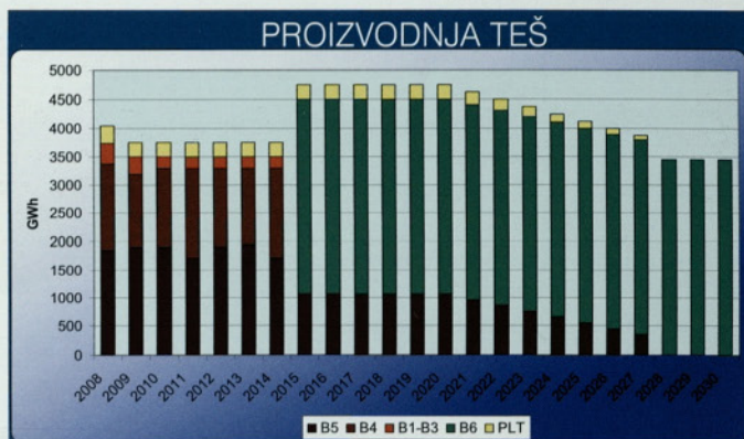
Prikaz sedanje in bodoče proizvodnje TEŠ do konca eksploatacije iz Premogovnika Velenje.
