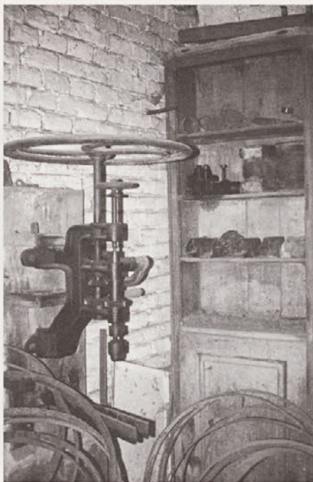
Ročni vrtalnik v Pernatovi kovačiji. (foto M. K., julij 1998).
