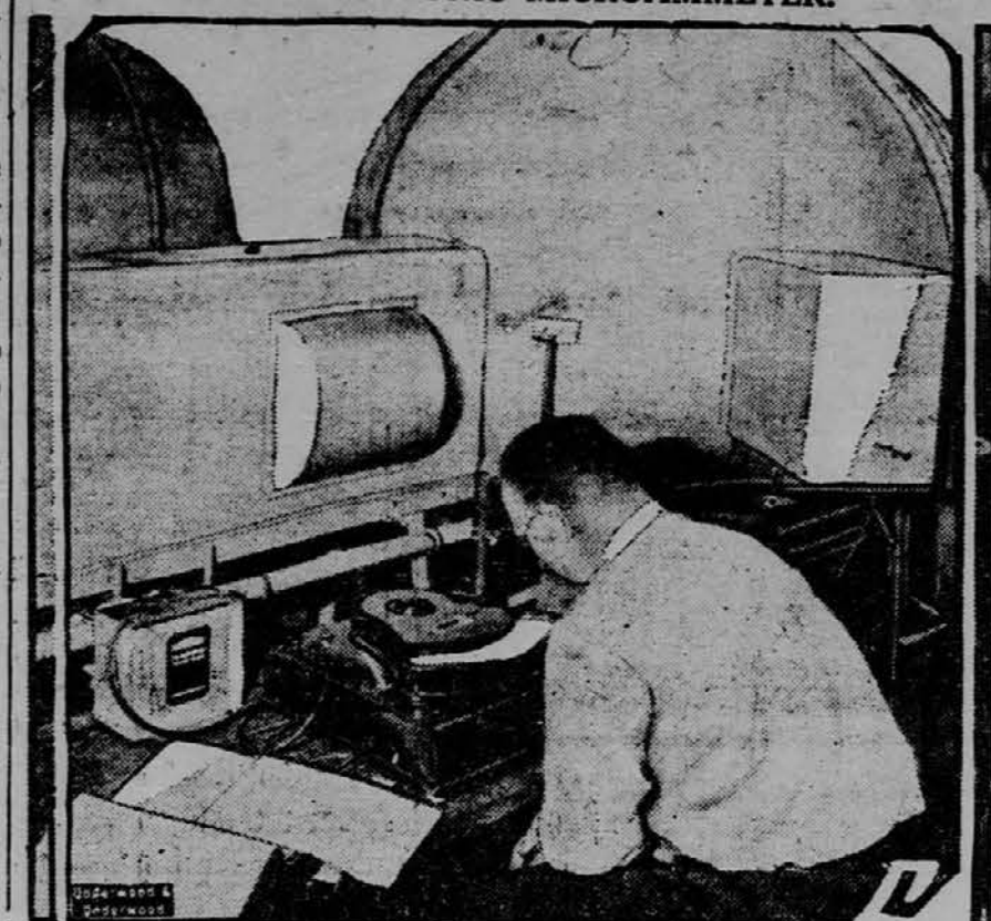
General Electric kompanija ima v svojem laboratoriju v West Lynn nov instrument, imenovan Thermionic Microammeter, s katerim preizkušajo žarnice, radio tube in druge električne vporabe.
