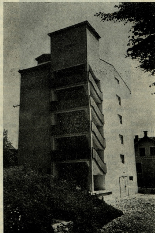
Tipska sušilnica za hmelj
