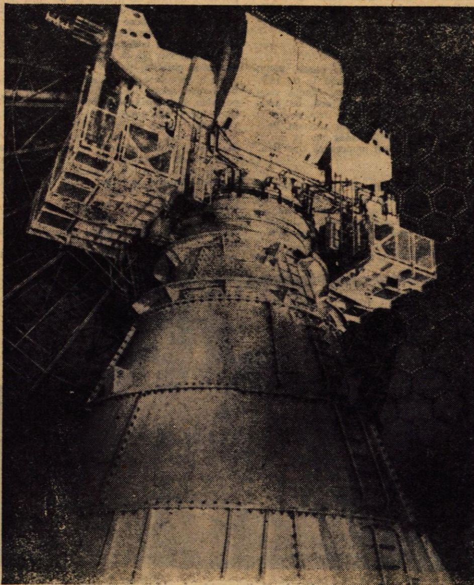
Nove radarske naprave, ki so jih Američani postavili na britanskem otočju. Naprave so zelo natančne in dovršene.
